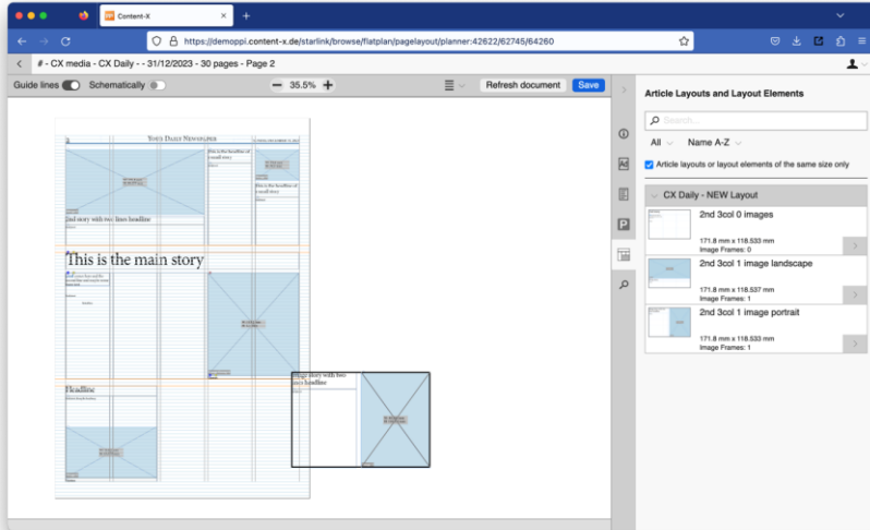
Web-basiertes Layout
